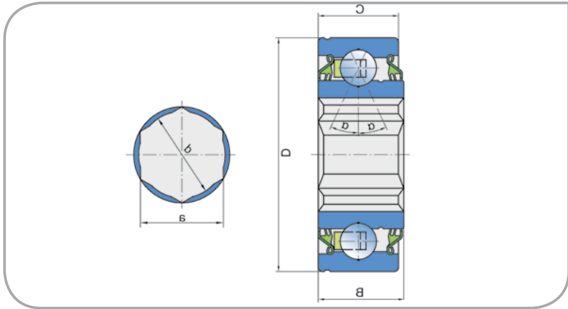
Dimensiones (mm)
