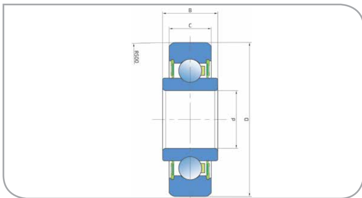
Dimensiones (mm)
