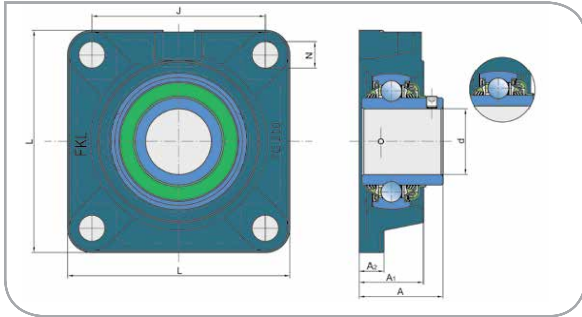
Dimensiones (mm)
